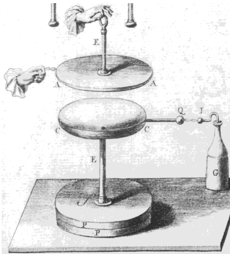
Figure 1. Volta's electrophorus with Leyden jar. From Scelta di Opuscoli (1775). 52
